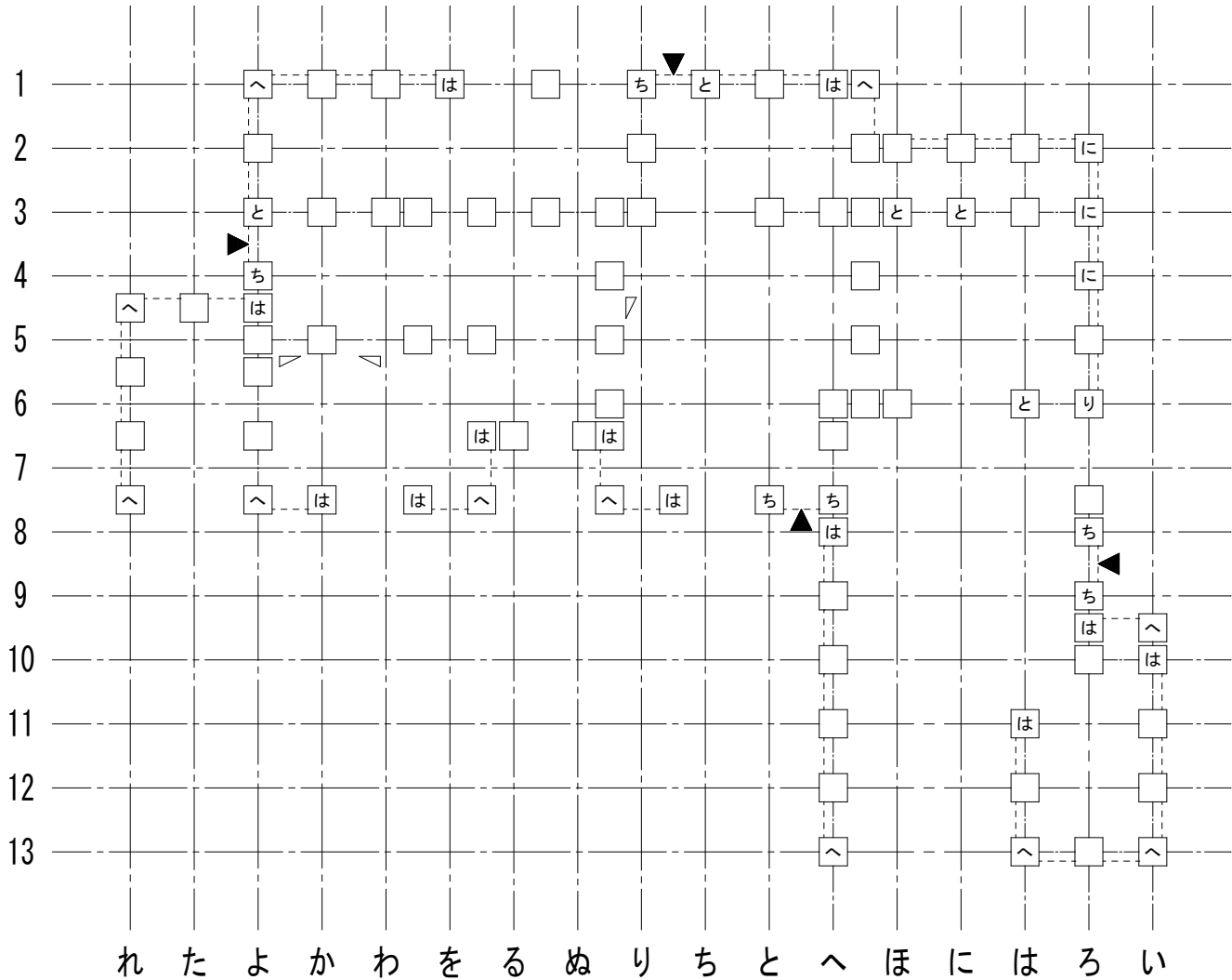
1階柱壁伏図
