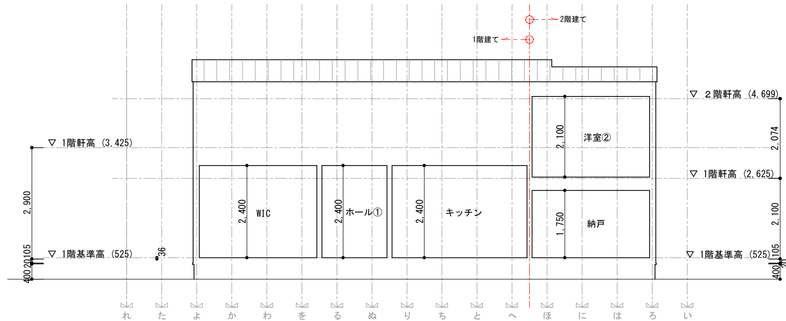
断面図(東西) S=1/100
