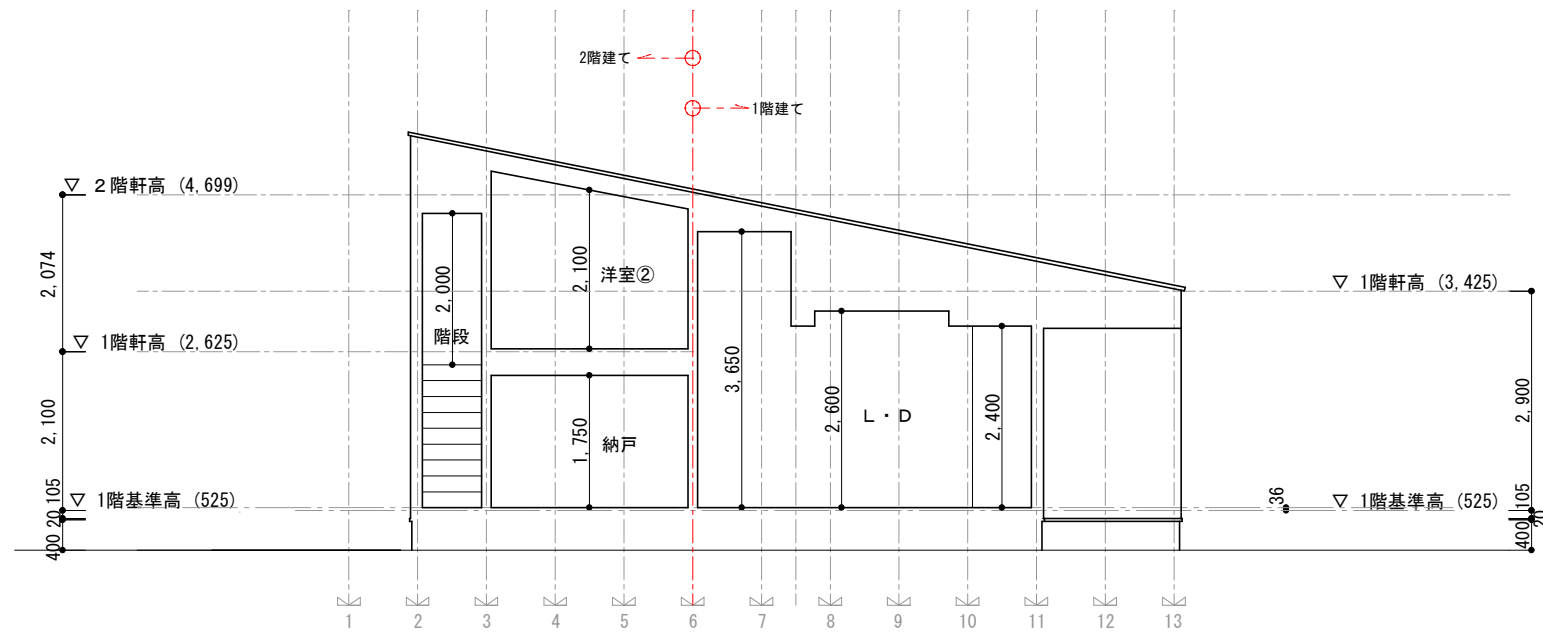
断面図(南北) S=1/100
