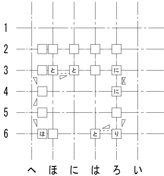
2階柱壁伏図
